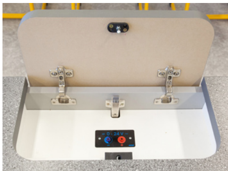
Trojlice s NN panelem v odklopu. Zdroj napětí pro NN panely
